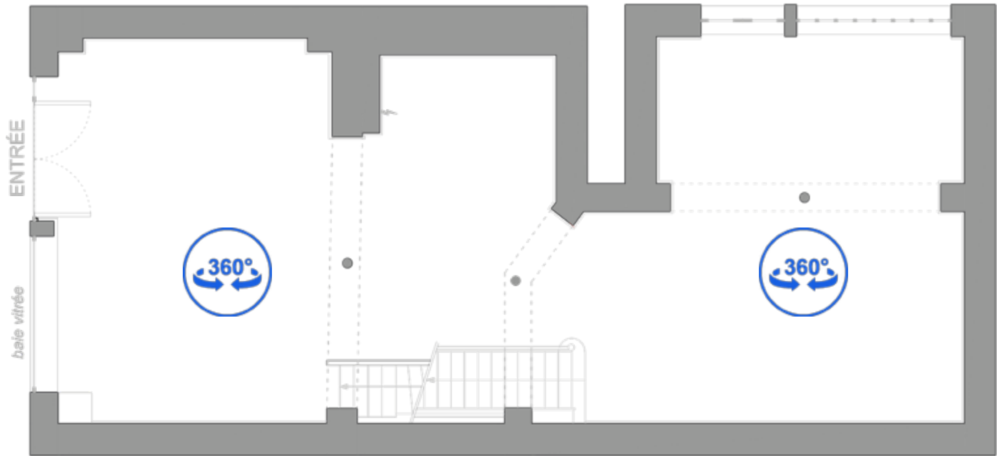
PLAN REZ-DE-CHAUSSÉE
